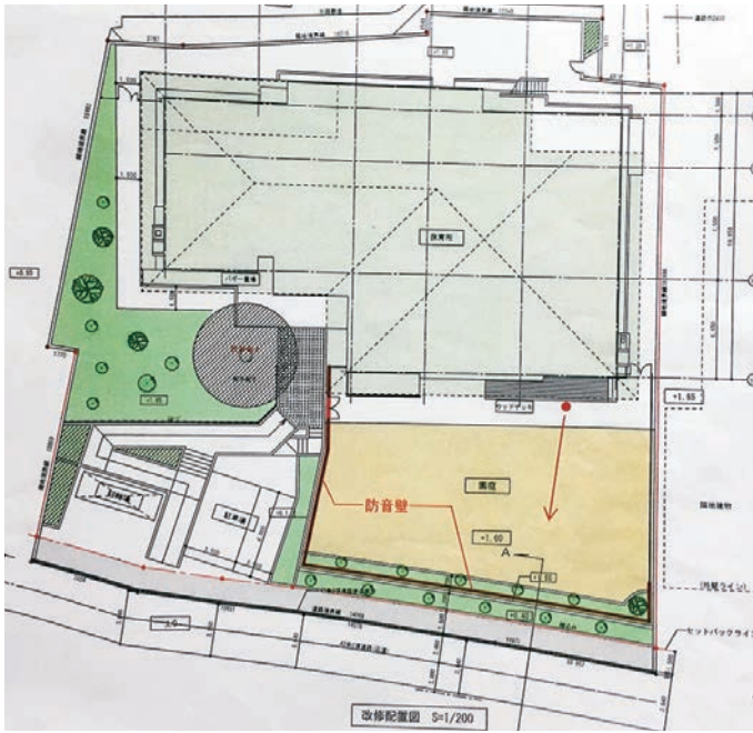
ふれあい館を改修し、新しくなる志茂保育園の平面図
